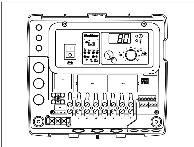
Kuva 25. Kaapelien reikäaihioiden paikat kotelon pohjaosassa Bild 25. Platser för kabelgenomföringarna i bottendelen av styrcentralen
